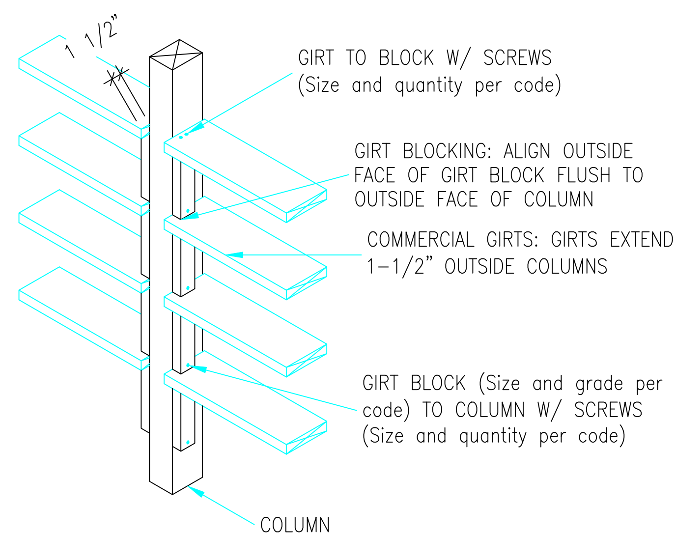
19-1 COMMERCIAL GIRT TO COLUMN S-5 SCALE: N.T.S.
