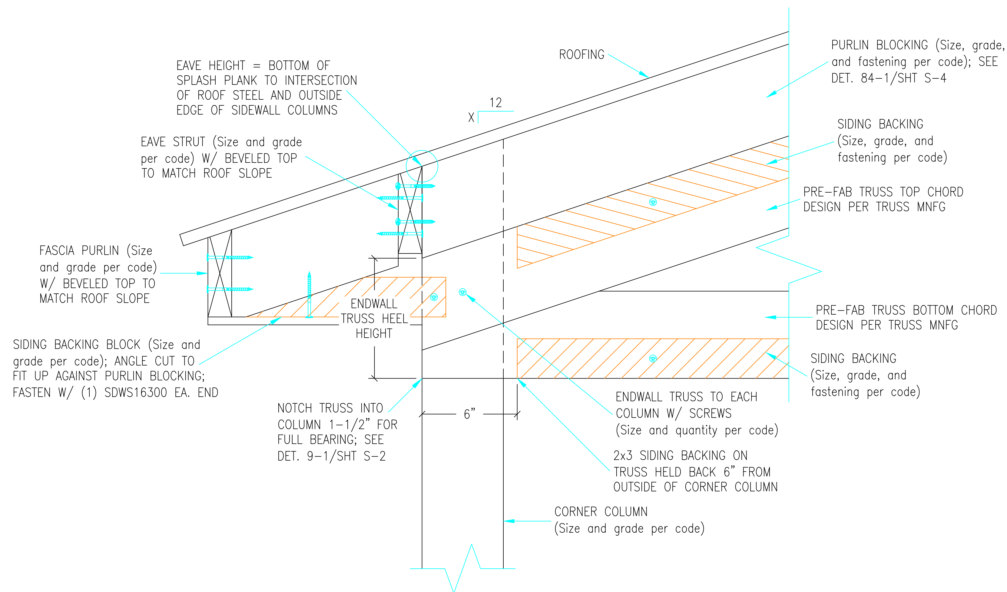
83-1 ENDWALL TRUSS TO COLUMNS S-4 SCALE: 2"=1'-0"
